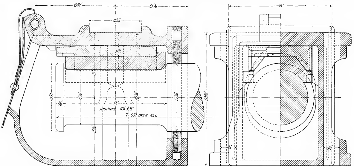
Fig. 5383. Longitudinal Section.
